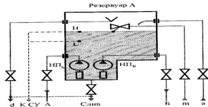
Схема противопожарного водоснабжения ВПВ или ВПВ, совмещенным с АУП, и/или с ХПВ, или с производственным водопроводом из одного пожарного резервуара (при наличии общего приямка для всех пожарных насосов)
