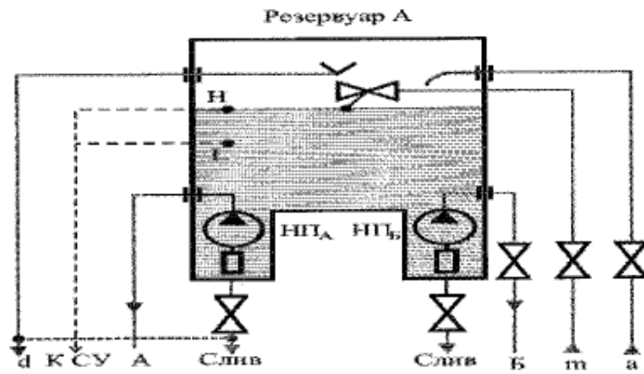
Схема противопожарного водоснабжения ВПВ или ВПВ, совмещенным с АУП, и/или с ХПВ, или с производственным водопроводом из одного пожарного резервуара (при наличии приямка для каждого пожарного насоса)
